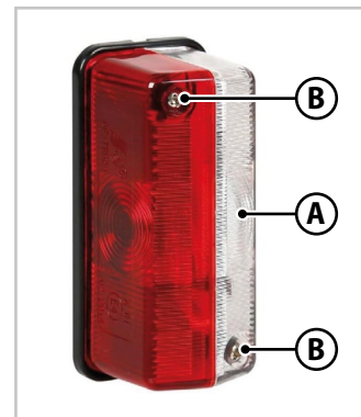
Fig.7.3 - Feux de gabarit latéraux
