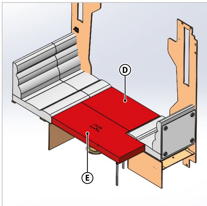
6. Mettre en place les coussins supplémentaires D et E .
