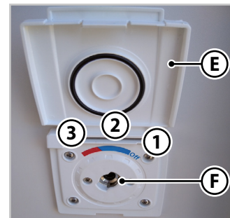
Fig.6.34 - Saída de engate do duche
